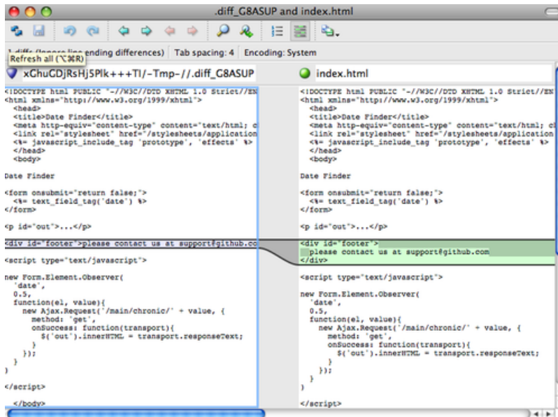
图 7-1: P4Merge。
